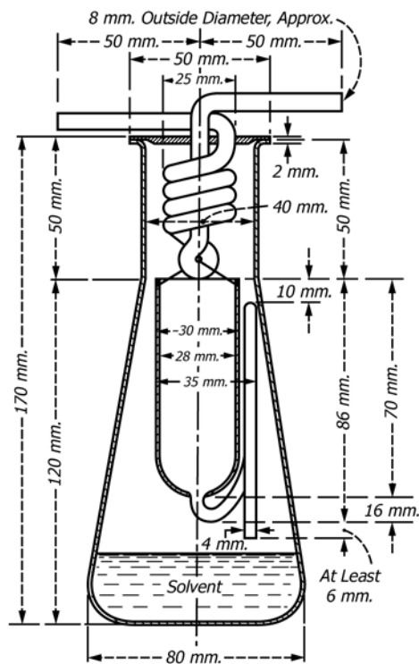
FIG. 1 Extraction Apparatus
