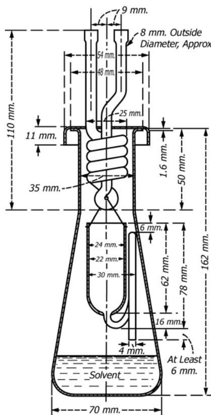
FIG. 2 Extraction Apparatus
