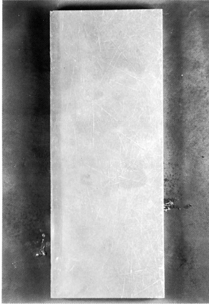
FIG. 16 Resin-Rich Edge
