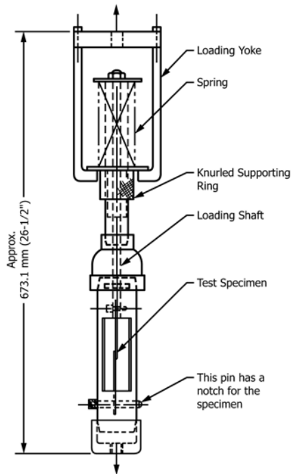
FIG. 1 Tension Creep Test Apparatus
