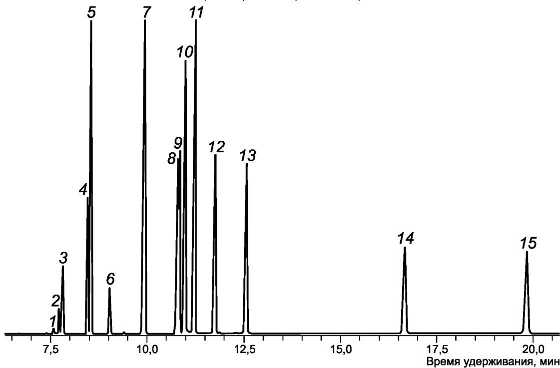
1 — метан; 2 — этен; 3 — этан + ацетилен; 4 — пропен; 5 — пропан; 6 — пропадиен; 7 — изобутан; 8 — изобутен; 9 — бутен-1; 10 — бутадиен-1,3; 11 — n -бутан; 12 — транс -бутен-2; 13 — цис -бутен-2; 14 — изопентан; 15 — n -пентан
