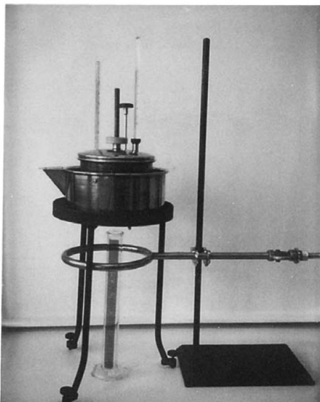
Рисунок 2 – Вискозиметр Энглера с мерным цилиндром вместимостью 50 см 3
