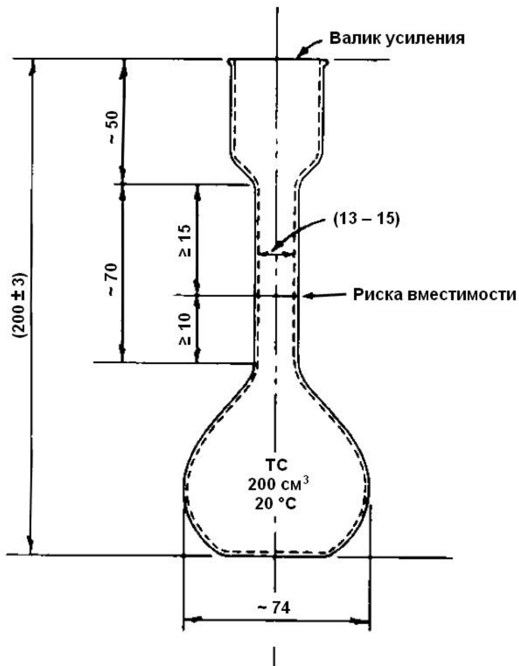
Рисунок 3 – Колба Кольрауша
