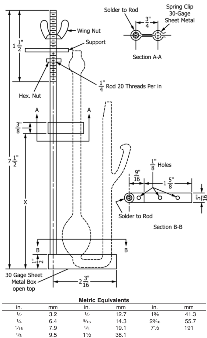
FIG. 3 Pycnometer Holder
