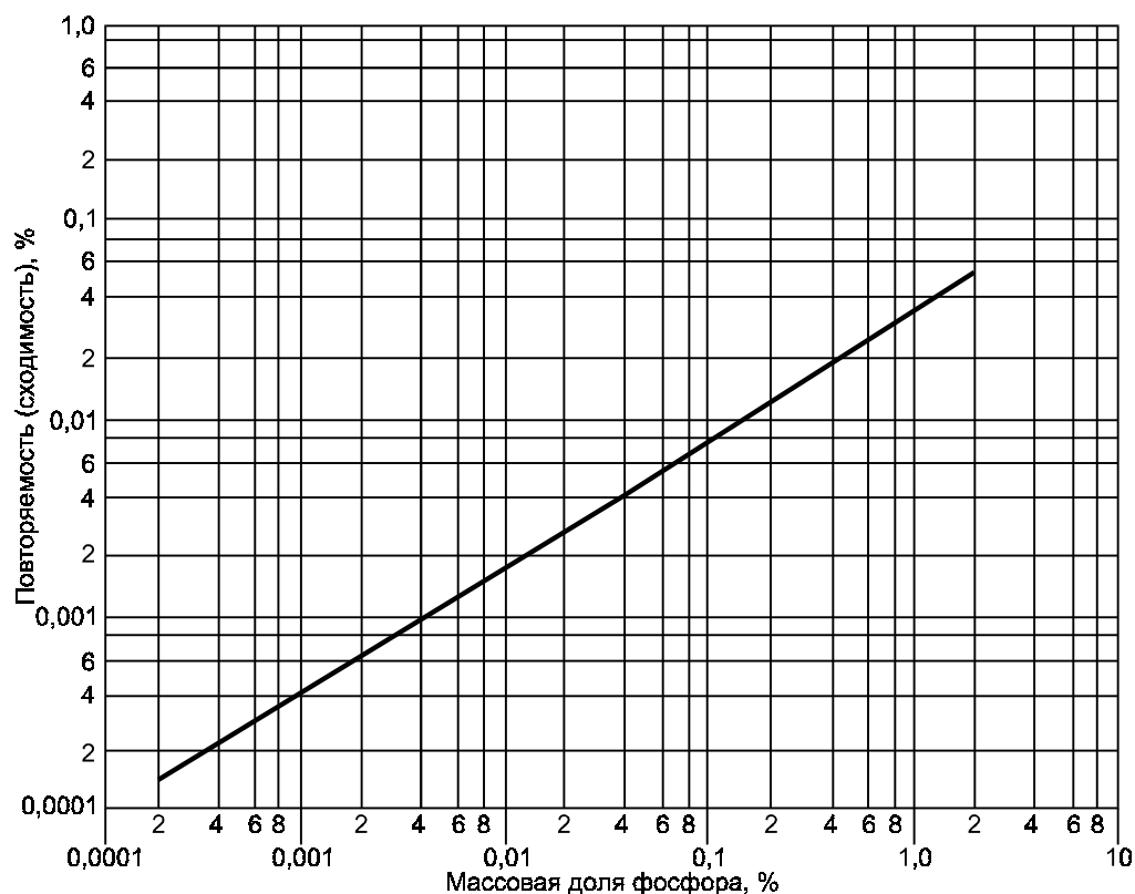
Рисунок 1 — Повторяемость (сходимость) фотометрического метода
