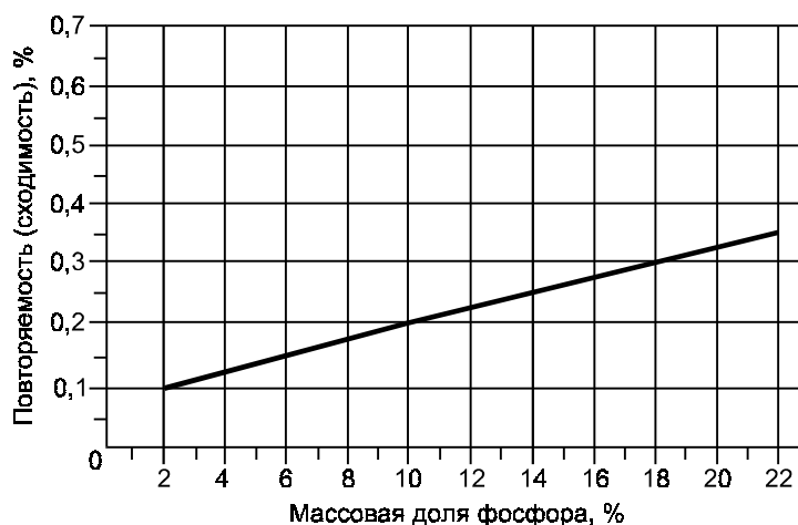
Рисунок 2 — Повторяемость (сходимость) гравиметрического метода
