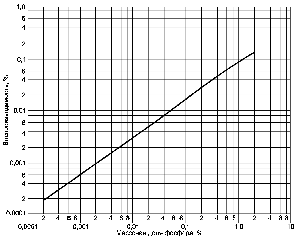
Рисунок 3 — Воспроизводимость фотометрического метода
